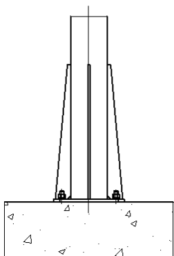
Mocowanie dolne przewodnicy A
