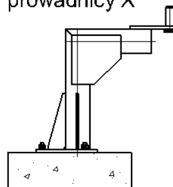
Mocowanie górne prowadnicy X
