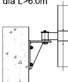
Mocowanie dolne A
